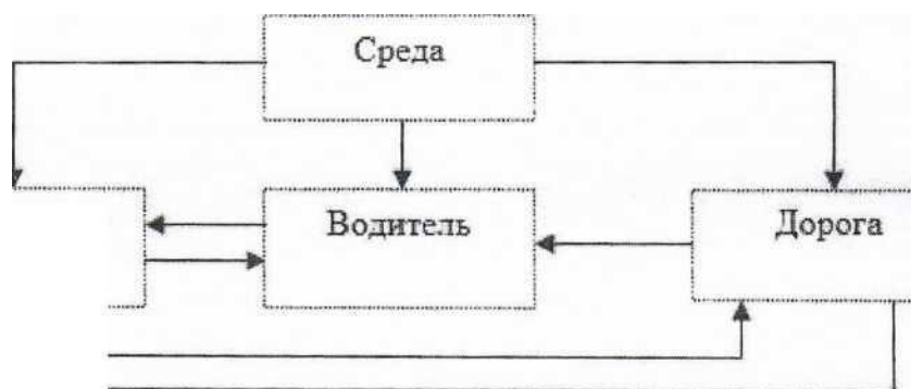
Структурная схема системы «водитель-автомобиль-дорога-среда движения»
